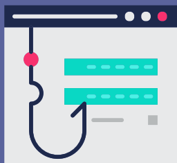
JEBAKAN PHISHING
